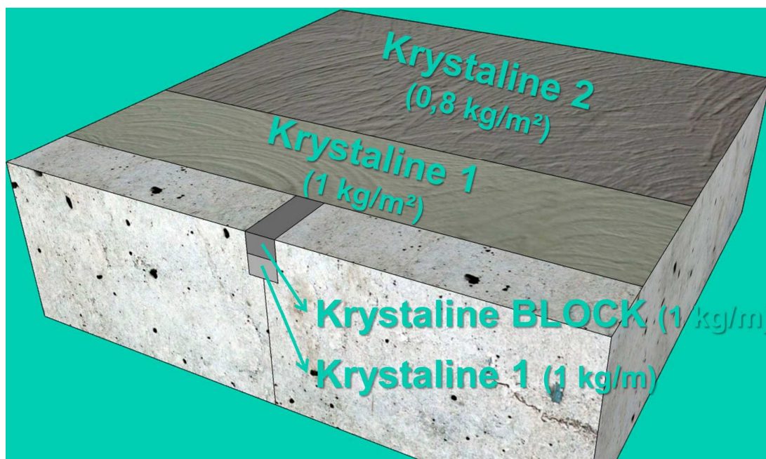
Rys.1. Przykład zastosowania zaprawy KRYSTALINE BLOCK / BLOCK F oraz układ warstw materiałów KRYSTALINE (bez czynnego przecieku wody).
